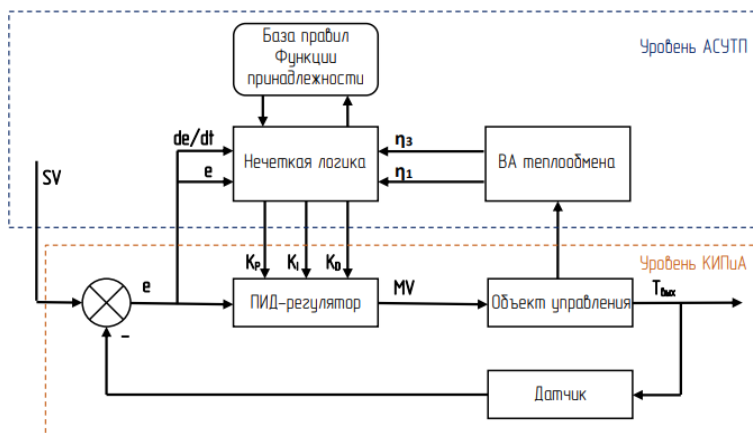
Рисунок 1 – Структурная схема предлагаемой нечёткой адаптивной системы автоматического регулирования температуры с ПИД-регулятором
