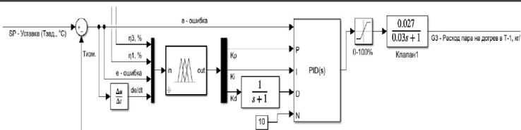
Рисунок 2 – Модель объекта с регулятором на базе нечеткой логики
