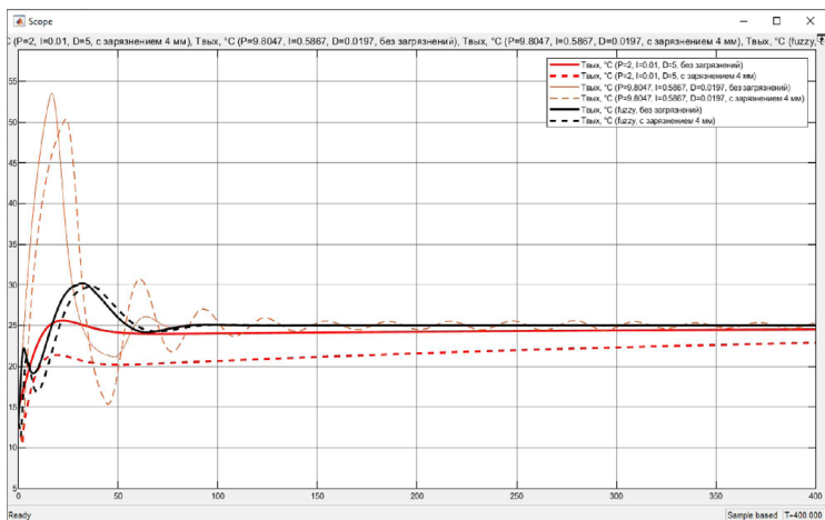
Рисунок 3 – Моделирование работы системы управления в пусковом режиме
