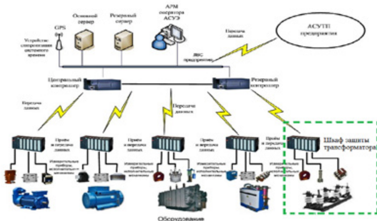
Сурет 2 – кәсіпорынның АСУТП құрылымындағы трансформаторды қорғау шкафы
