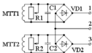
Сурет 4 – қорғаныс шкафына МТТ электр қосылымының схемасы 4-суретте R1 айнымалы резисторлары мен C1 конденсаторларының
