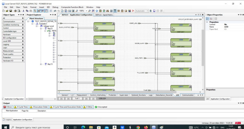
Рисунок 7 – В инструменте конфигурации логики переменная «TP_CLOSED» подключен к светодиоду 10.
